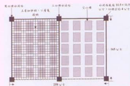
圖1. 堆肥箱底部平面圖
