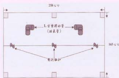
圖2. 堆肥箱頂部平面圖
