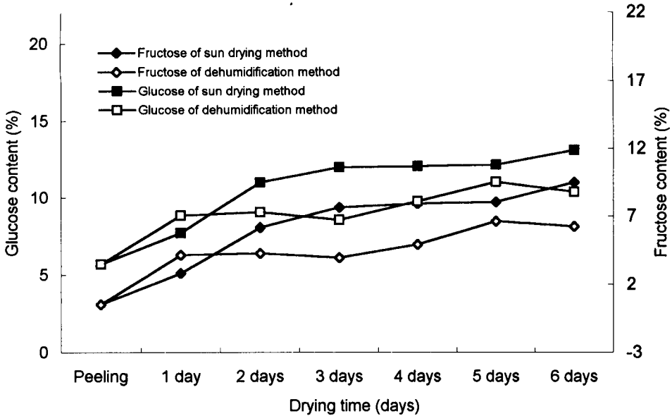
圖 7. 自然日曬法與除濕乾燥法製造柿餅期間葡萄糖與果糖之變化
