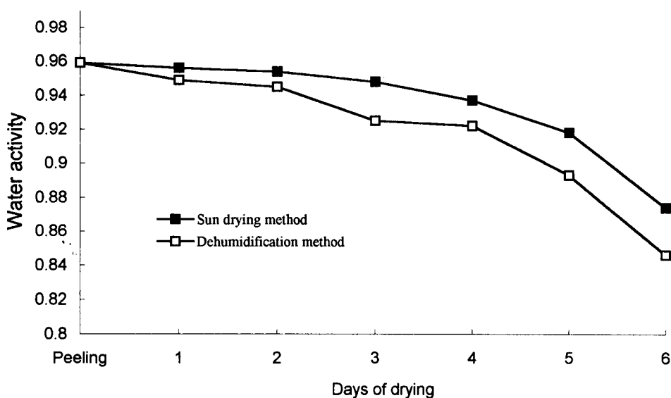
圖 9. 自然日曬法與除濕乾燥法所製成柿餅之水活性比較
